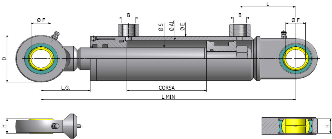
CILINDRO DOPPIO EFFETTO TIPO SDC
