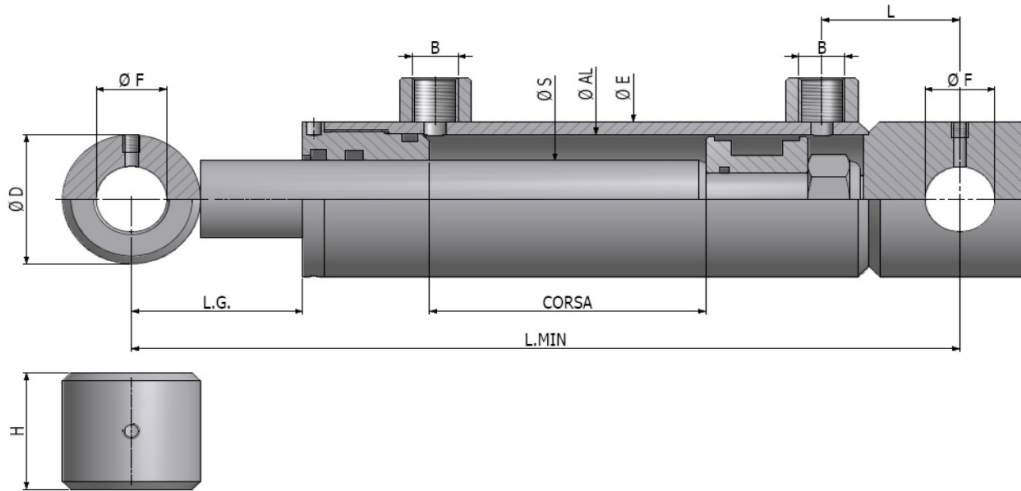
CILINDRO DOPPIO EFFETTO TIPO FDA
